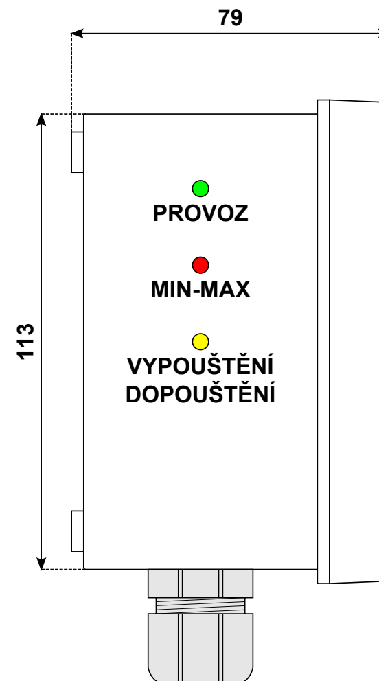
Snímač hladiny MAVE 2-S3
